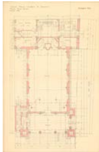
10. Tempio Valdese, planimetria piano terra scala 1:50, 1923. Archivio privato Tempio Valdese, Palermo.
