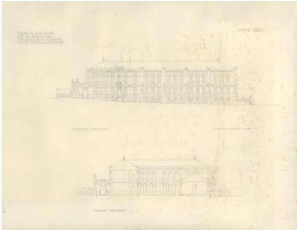
10. Antonio Lo Bianco, Concorso per edificio scolastico, via Fratelli Cairoli, Mantova, 1911, alzato del prospetto principale e sezione trasversale, 1/200, matita su cartoncino, 516x655 mm, s.d.; denominazione del progetto, intitolazione del disegno a matita. Tavola contrassegnata dal motto “ Spes ” (Archivio Progetti Lo Bianco, Collezioni Scientifiche, Dipartimento di Architettura, Università degli Studi di Palermo)
