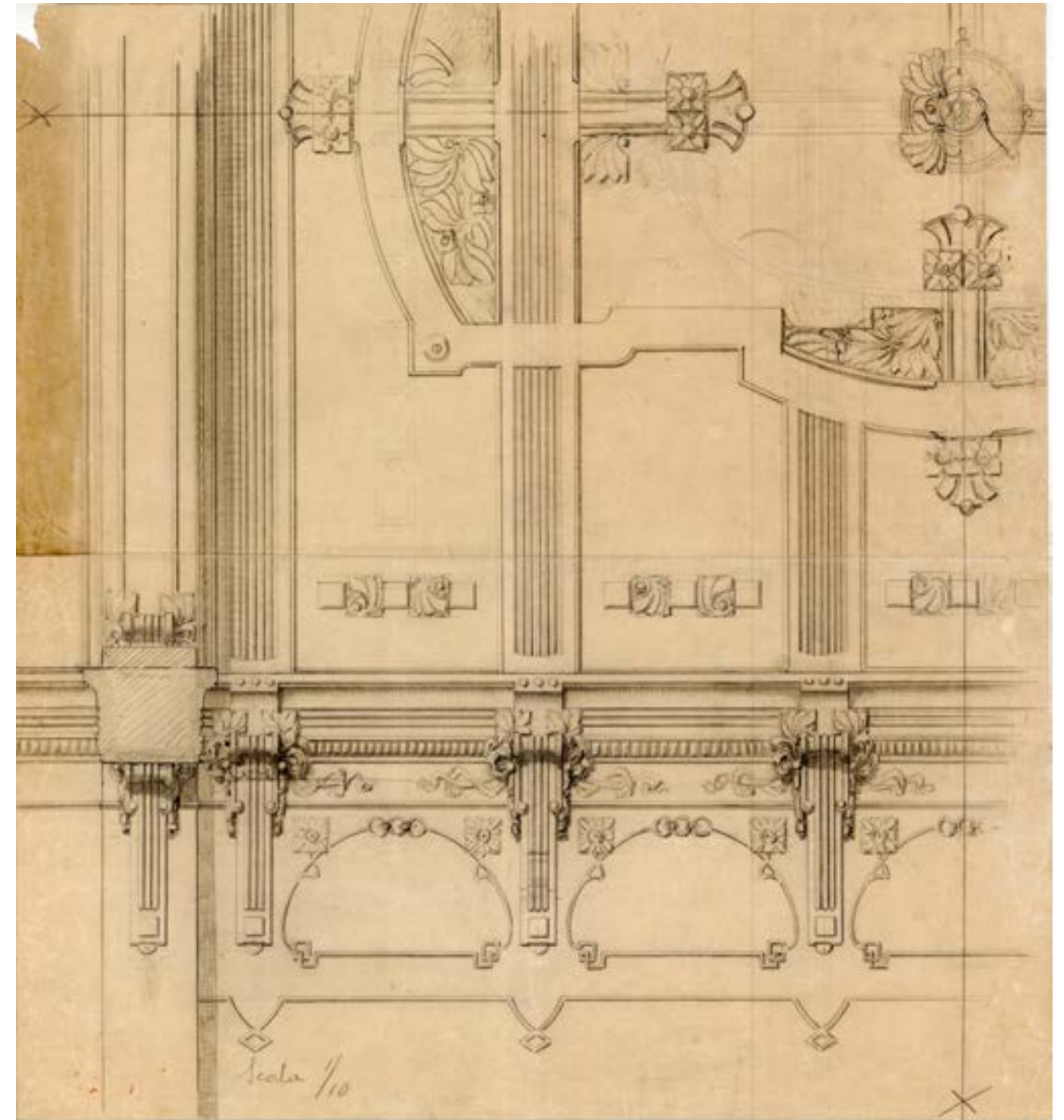
DITTA F.LLI MUSSO E PAPOTTI, Bozzetto per la cornice delle pareti dello scalone, s.d. [1905-07], PoliTo, DIST-APRi, Fondo Carlo Musso, MC 55.
