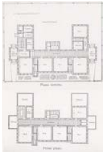
4. Nicolò Mineo, Scuola elementare Francesco Saverio Cavallari, corso dei Mille, Palermo, 1904-1907, pianta del piano terra e del primo piano, s.d., quotato; destinazioni degli ambienti (da «L'Architettura Italiana», VIII, n. 3, 1913, p. 46)
