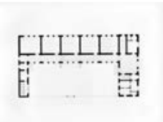
1. Ernesto Basile, Scuola elementare tipo per la Sicilia, (1895), pianta del piano terra con arredo delle aule, matita e china su cartoncino, 555x697 mm, (1895), s.t. Nel verso: studi di carpenteria metallica a matita; annotazioni, conteggi a matita (Archivio Disegni, Dotazione Basile, Collezioni Scientifiche, Dipartimento di Architettura, Università degli Studi di Palermo)
